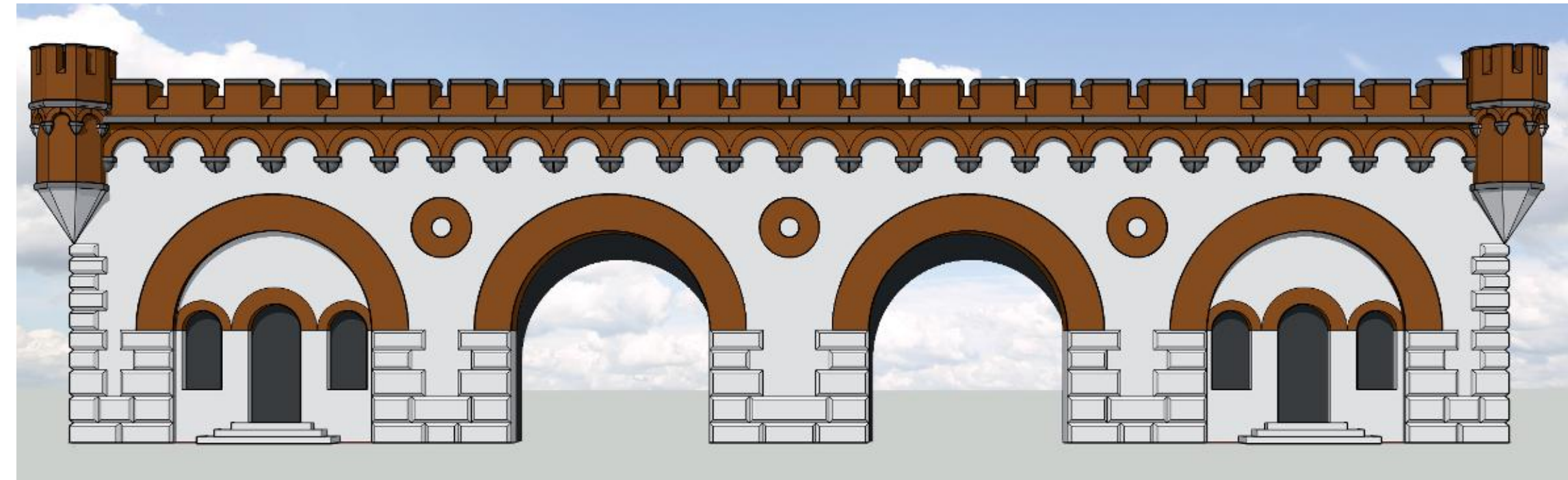
Blaubeurer Tor, Stadtfassade, CAD-Modell des ursprünglichen Zustands
